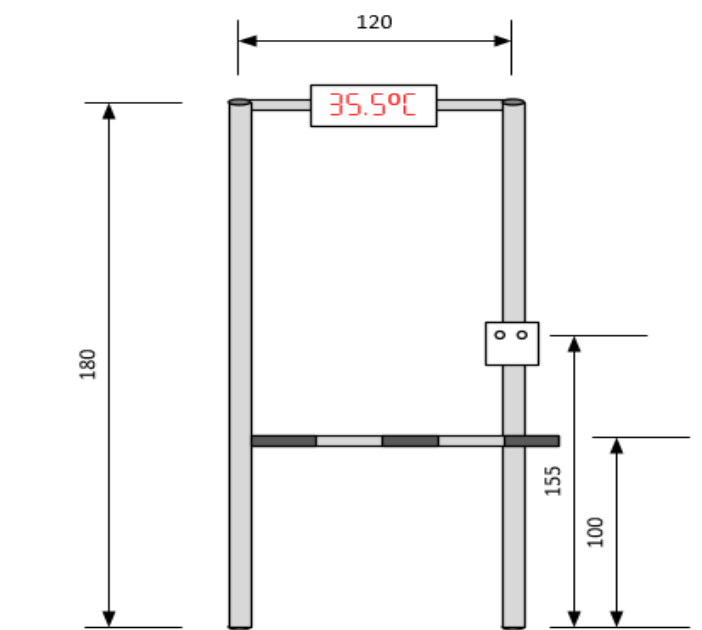
Gambar 1. Rancangan Pintu Portal
