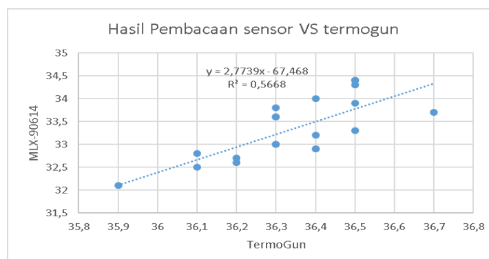
Gambar 5. Variabel kalibrasi sensor
